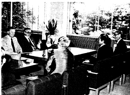
理事長・学長を表敬訪問（5月9日 左：ジャスミン氏、右：デイトン氏）
